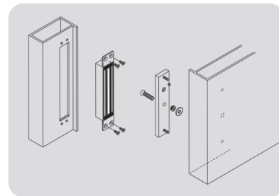
Fixation classique par vis Plaques de montage fournies
