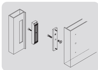
Fixation affleurante anti vandale par vérin
